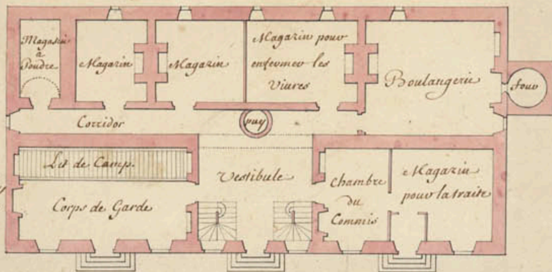
Plan de l'Etage au Rez de Chaussée.
